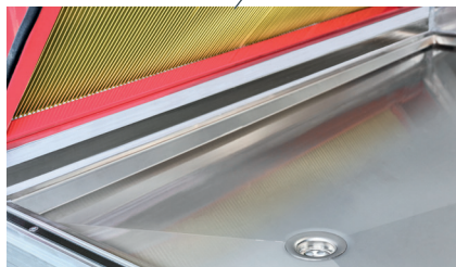
Rostfreie V2A-Tropfwanne mit allseitigem Gefälle (Ausführung nach VDI 6022).
